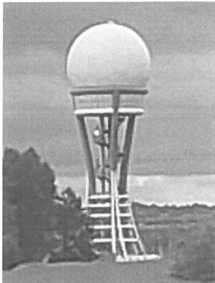
Widok obiektu wraz z zainstalowanym zespołem antenowym
